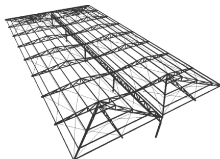
Projeto 3D quatro águas
