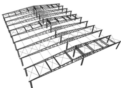
Projeto 3D com uma coluna no meio
